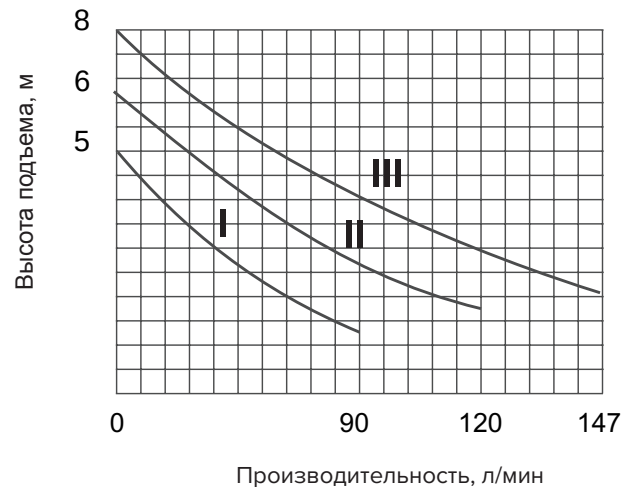
Рисунок 3 — График соотношения высоты подъема и производительности для насоса циркуляционного I-TECH 32/8/180
