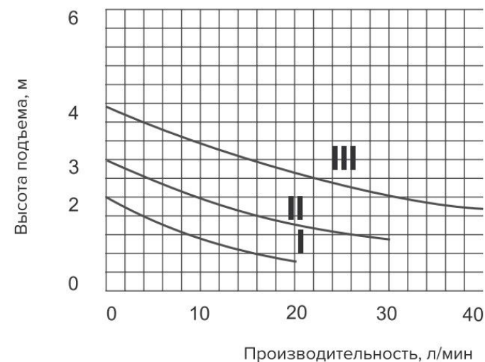
Рисунок 1 — График соотношения высоты подъема и производительности для насоса циркуляционного I-TECH 32/4/180
