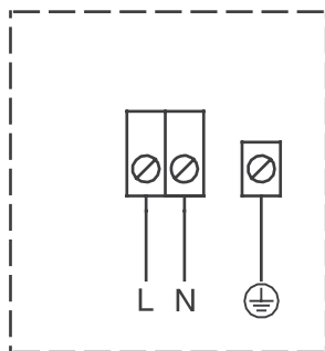
Рисунок 5 — Схема электрическая
