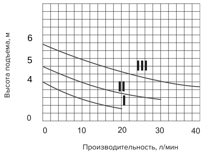
Рисунок 2 — График соотношения высоты подъема и производительности для насоса циркуляционного I-TECH 32/6/180
