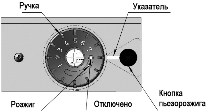
Рис. 10. Элементы управления на газовом клапане котлов Torino 7,5-20
